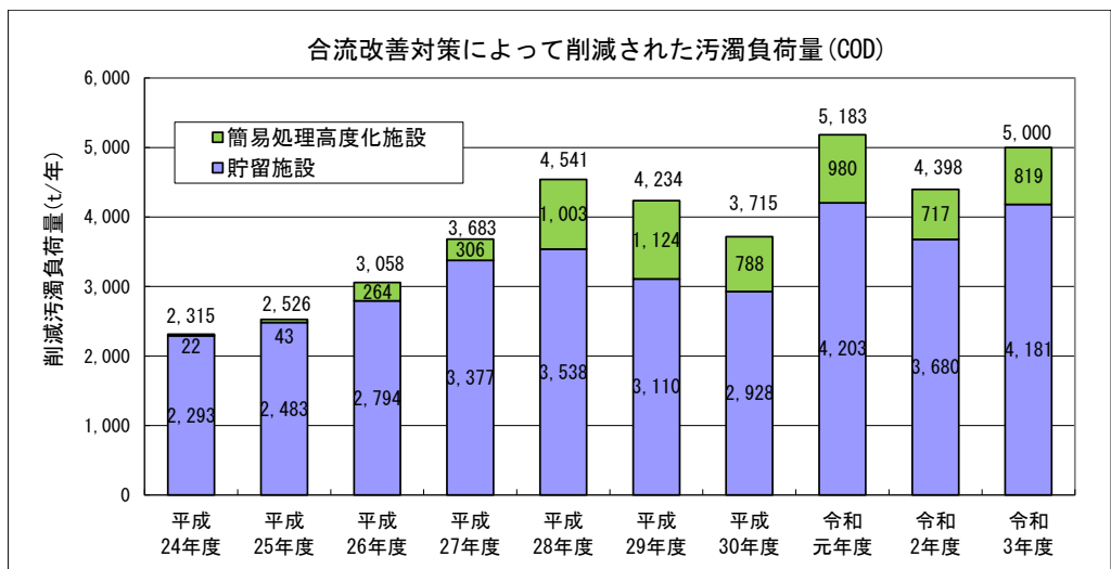
図 A3-3 削減汚濁負荷量の推移
