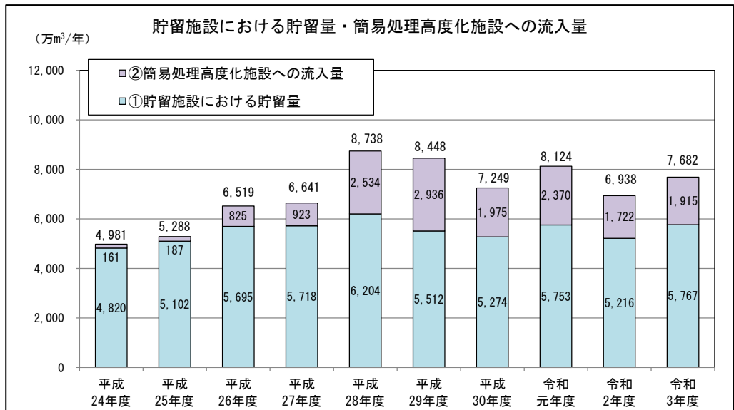
図 A3-5 貯留施設における貯留量・簡易処理高度化施設への流入量の推移
