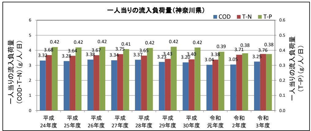
図 D2-3 都県別の下水処理施設から排出される一人当たりの流入負荷量
