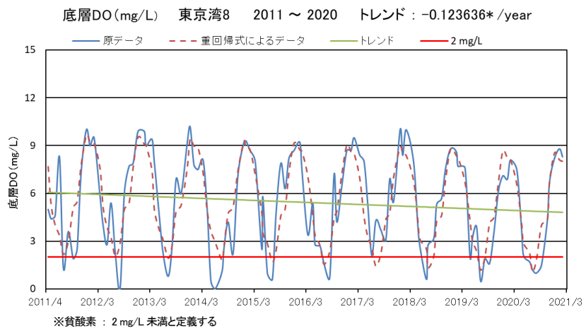
図 B4-2 DO (底層) (mg/L) の時系列変化および重回帰分析結果 (東京湾 08)
