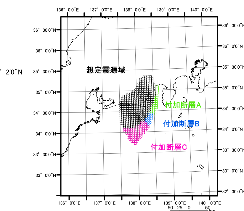
想定震源域と付加断層の位置
